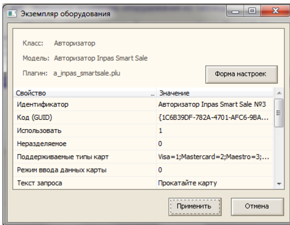
Рис. 6 «Список свойств авторизатора»
