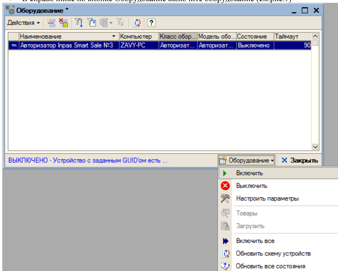
Рис. 9 «Справочник «Оборудование»»
