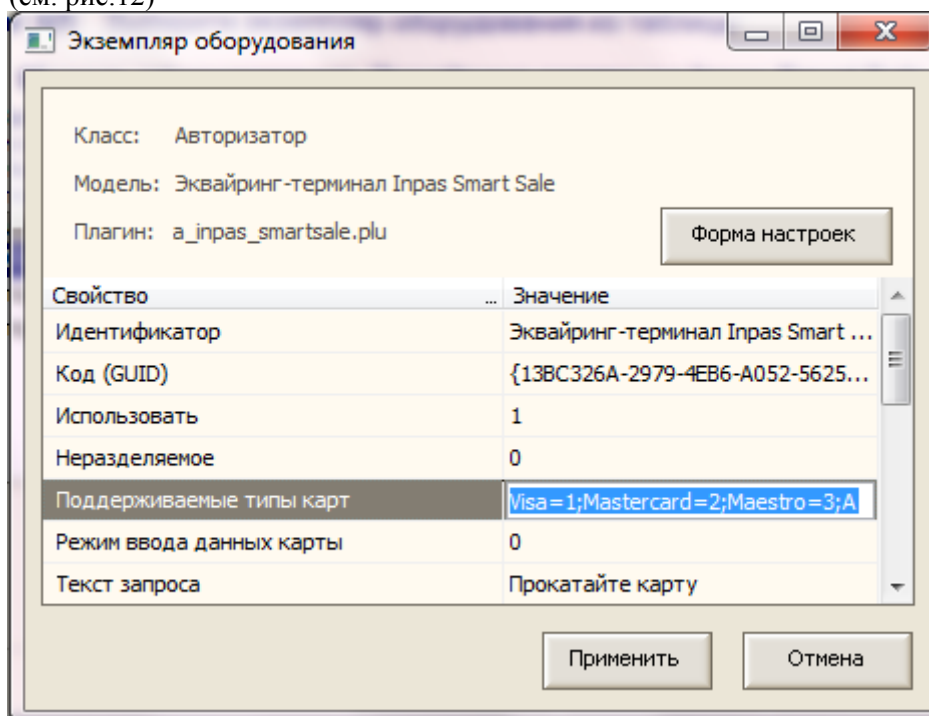
Рис.10 «Настройка Наименования типов платежных карт в настройках авторизатора» Настройка типов оплат в Справочнике «Типы платежных карт»
