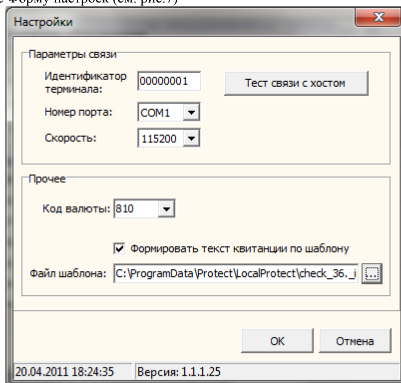
Рис. 7 «Настройки авторизатора»
